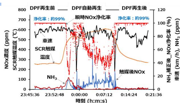
図3 実路走行時における尿素 SCR 触媒の瞬間 NOx 浄化率の変化
